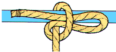
Slipstek
